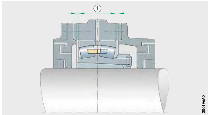
Figura 3 Soporte en ejecución de apoyo libre
