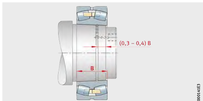
Figura 22 Anchura recomendada para las ranuras de aceite
